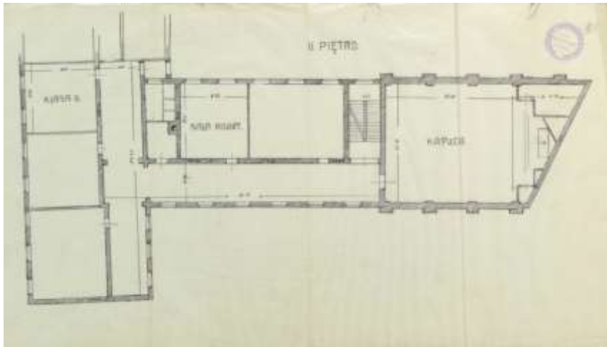
План третього поверху (добудова)
